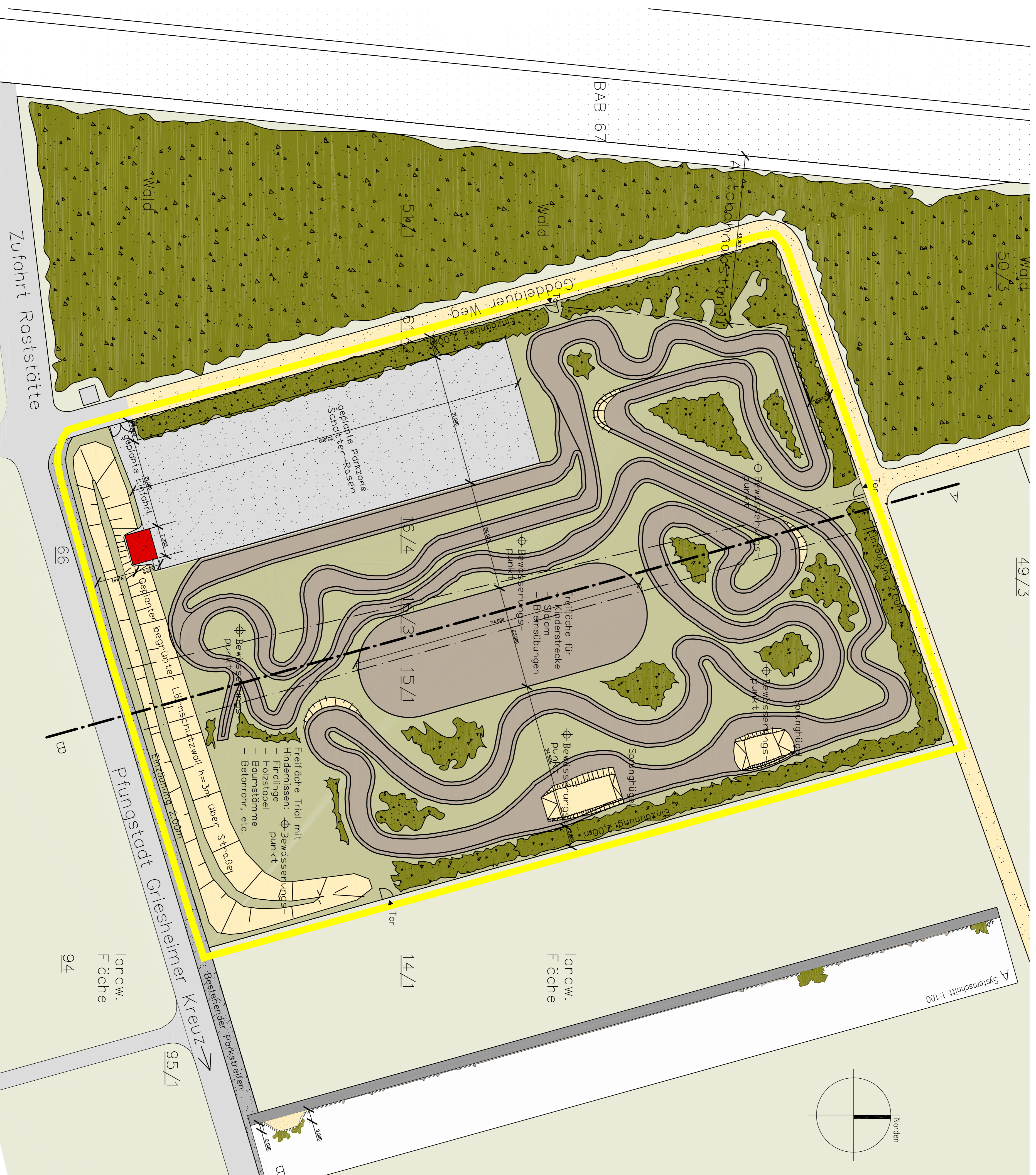
Lageplan 1:2000
